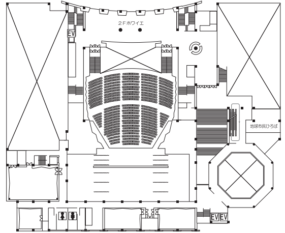
長崎ブリックホール 2階全体図
